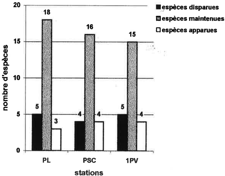
Fig. 1. Evolution temporelle de la richesse spécifique en Ephéméroptères du Volp entre 1963 et 2002 : espèces disparues, maintenues et apparues aux trois stations.
