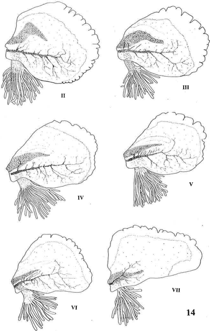
Pl. IV : structures larvaires au dernier stade de R. kimminsi .
