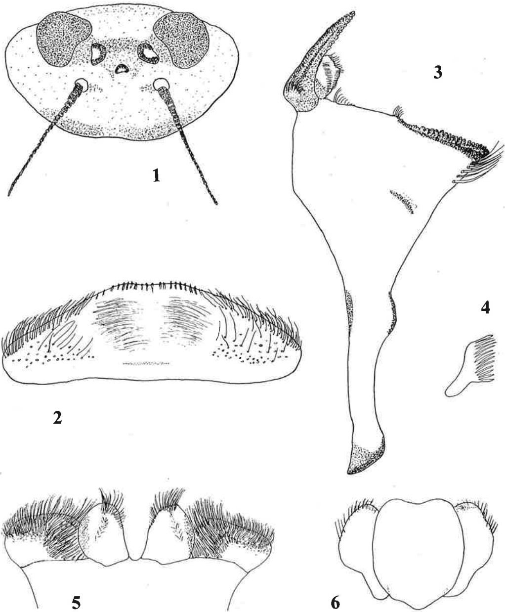
Pl. I : structures larvaires au dernier stade de R. kimminsi .
