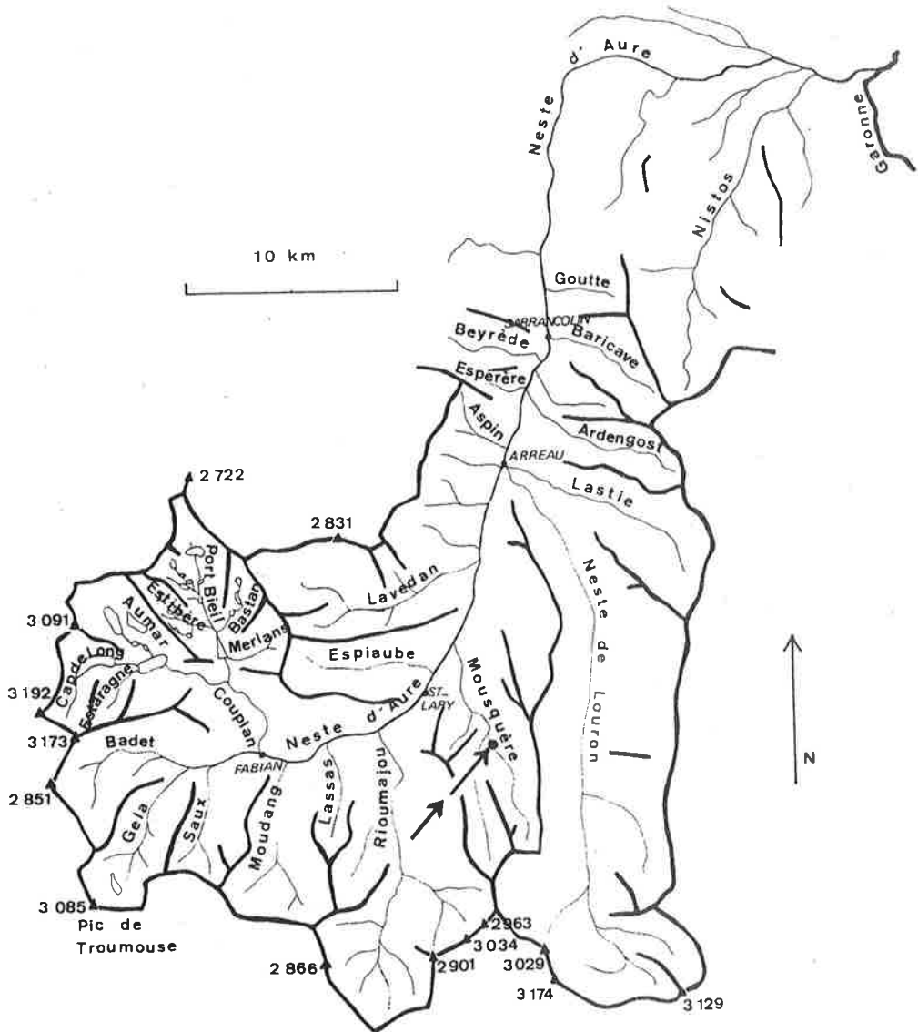
Carte 1. La vallée d'Aure : réseau hydrographique et lignes de crêtes (d'après H. Décamps). Flèche : Locus typicus.
